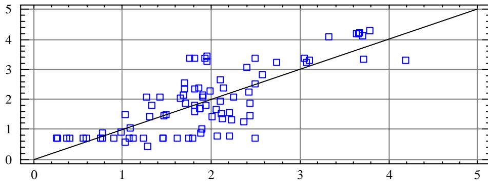
Ln (Ni)
