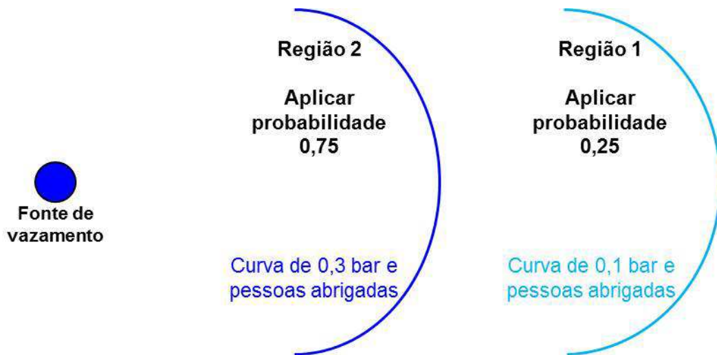
Figura 13 – Representação das regiões de probabilidade de fatalidade associadas aos valores de referência para o efeito de sobrepessão
